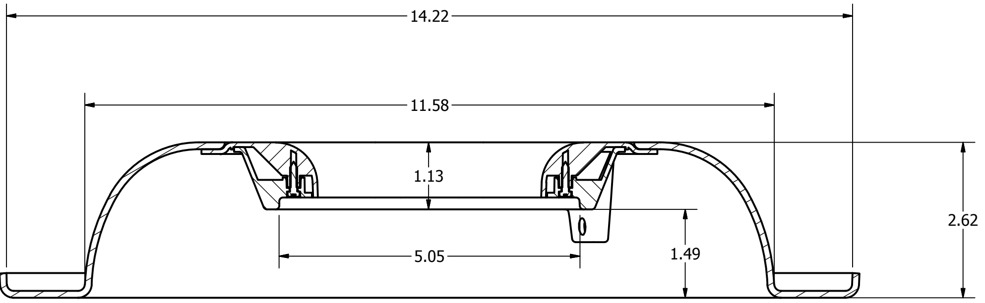
SECTION A-A
